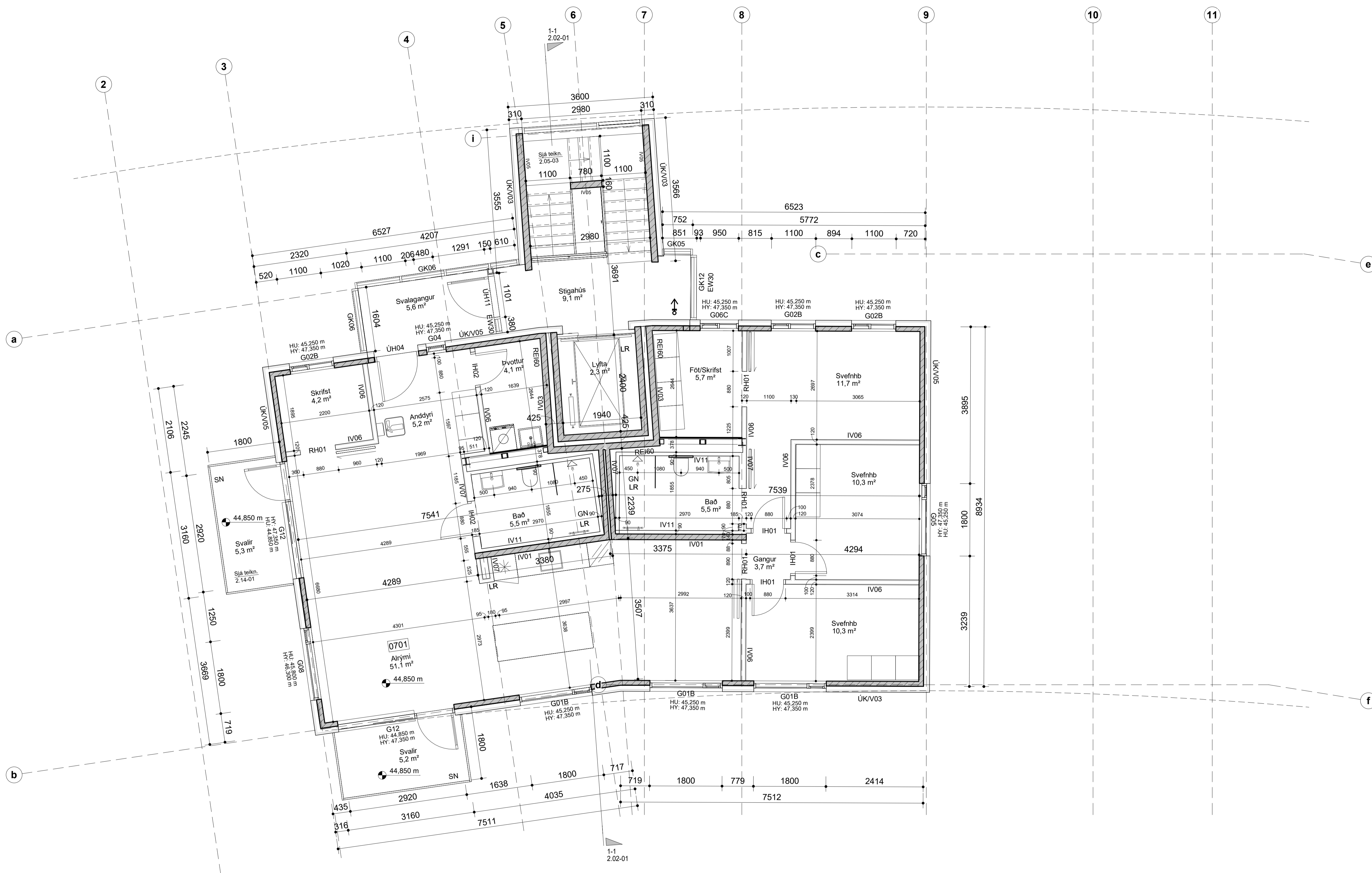
7.hæð - Verk. hús 6, hluti 1/2 mkv: 1 : 50
