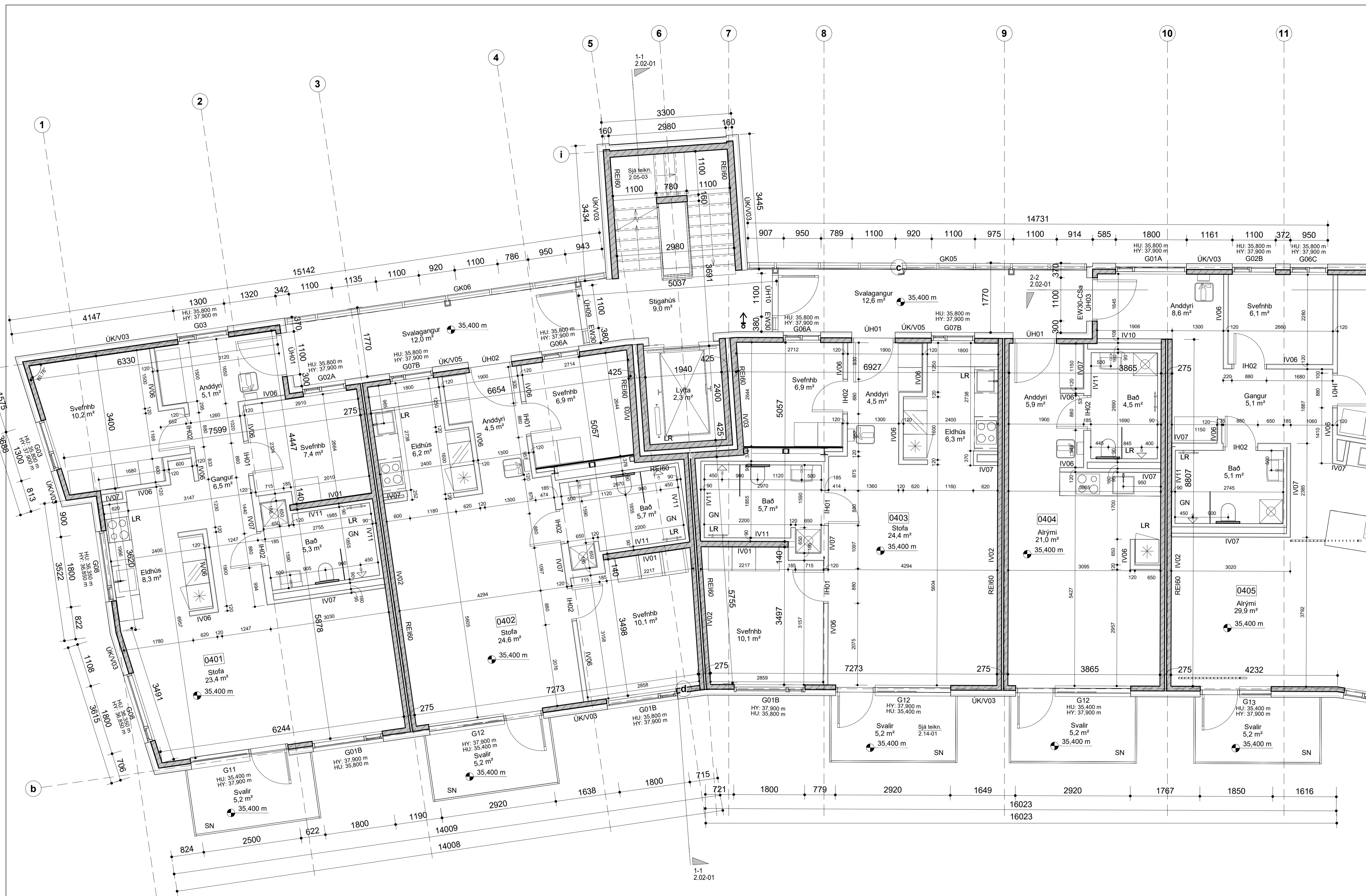
4.hæð- Verk. hús 6 - hluti 1/2 mkv: 1 : 50
