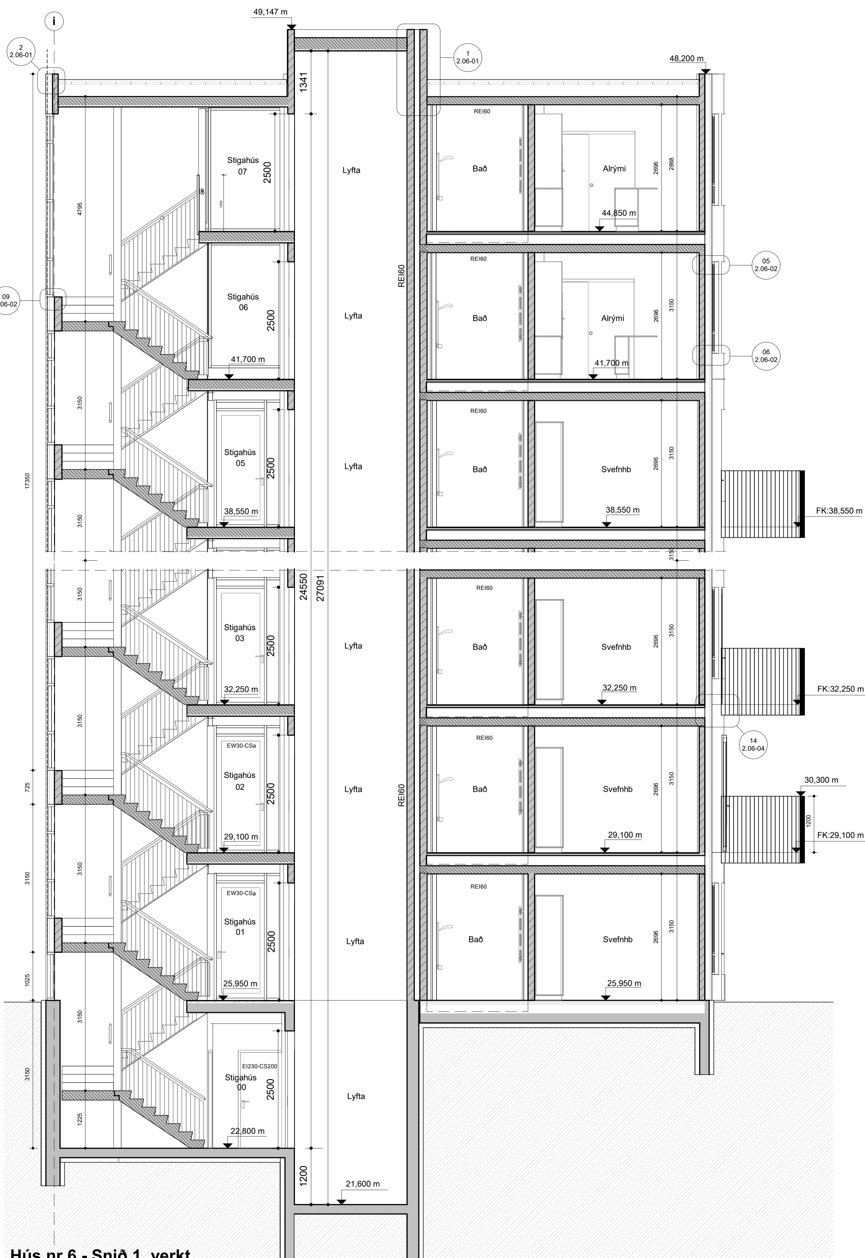
Hús nr 6 - Snið 1, verkt. mkv: 1 : 50
